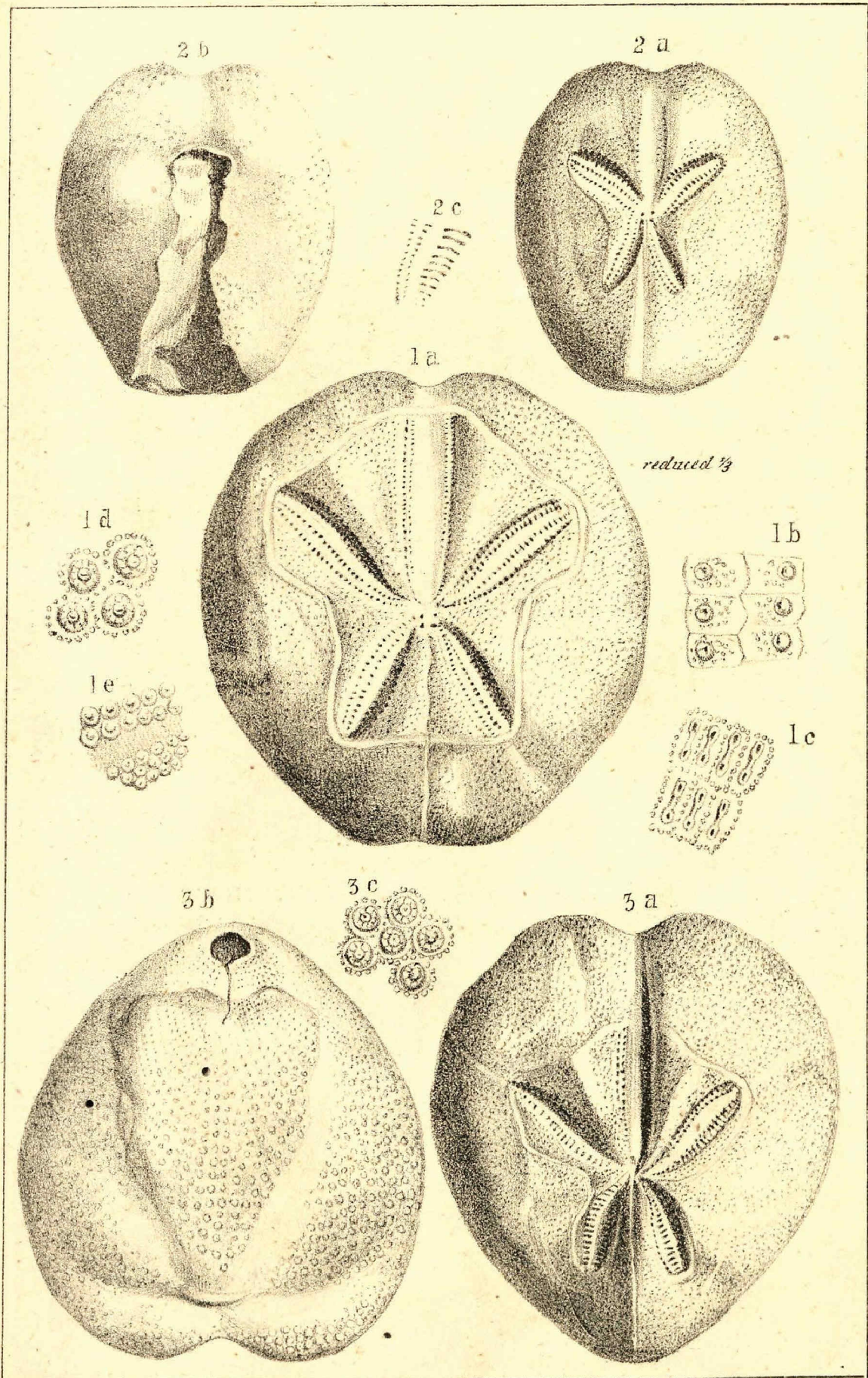
1 a-e Brissopsis Duciei , Wright 2 a-c Brissopsis crescenticus , Wright 3 a-c Schizaster Desori , Wright
