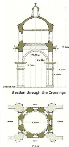
Cross-section tal-koppla mill-pilastru maġġuri (fuq) u pjanta tal-bażi ottagonali tal-koppla (isfel). (Hajr lil Joseph Spiteri)
