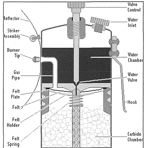
L-istruttura ta' lampa tal-idejn li taħdem bl-aċitilena. L-istess kunċett kien jintuża fit-tankijiet il-kbar li fihom kien jiġi prodott il-gass tal-aċitilena
