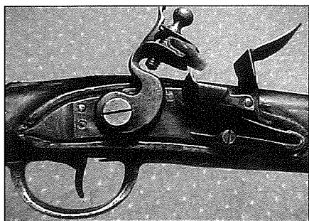
Fig. 1. Il-Mekkanizmu tal-Grillu ta' Xkubetta taż-Żnied 9 (i.e. Flint-Lock Musket )
